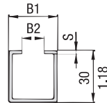
Tragschiene TS-30
